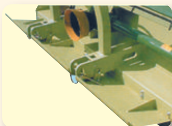
ACCESSORIO/ ACCESSORY/ACCESSOIRE/ ZUSATZ Convogliatore per sarmenti. Branches blade conveyer. Lame d'acheminement des sarments. Spezielle Front-Metallplatten zur Zuführung des Schnittgutes zum Mulch-Rotor.
